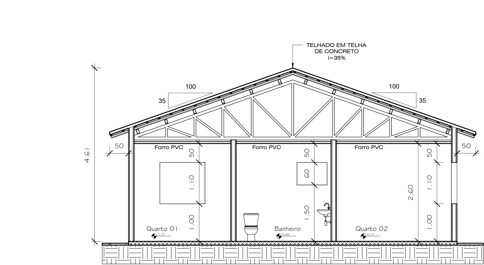
Corte B 1 : 50
