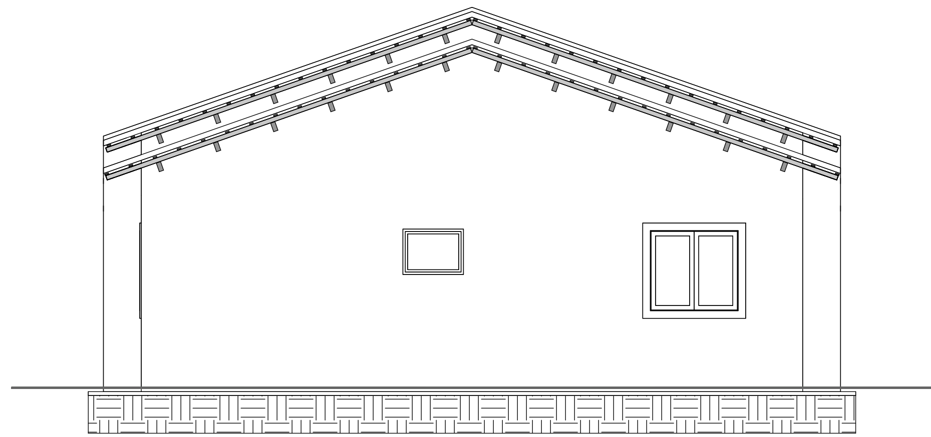
4 Elevação Lateral 1 : 50
