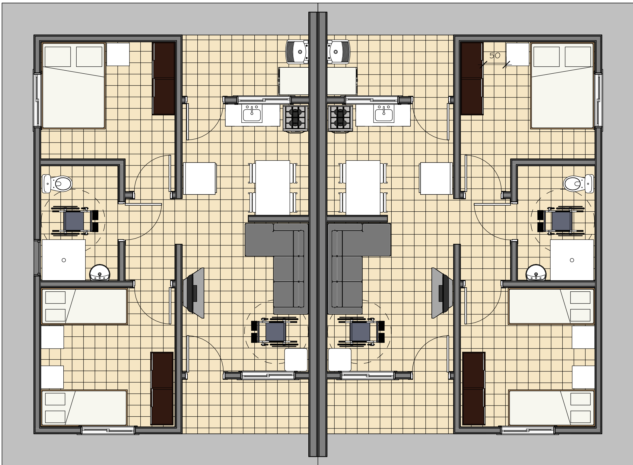
2 Planta Baixa - Layout humanizado 1 : 50
