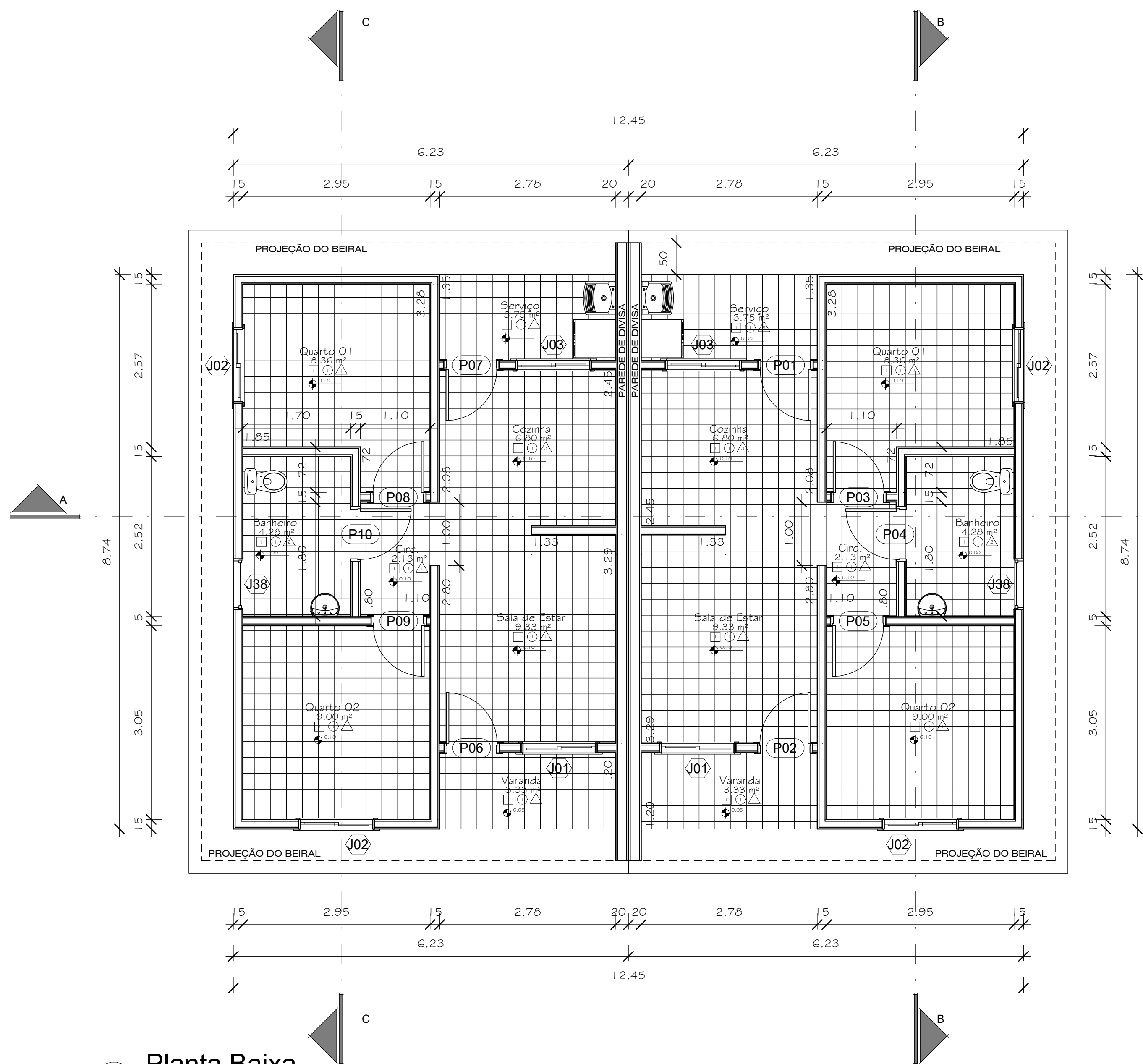
1 Planta Baixa 1 : 50
