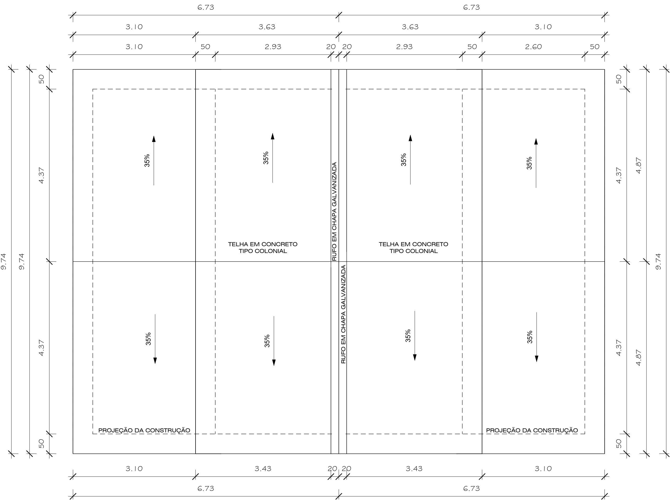
1 Planta de Cobertura 1 : 50
