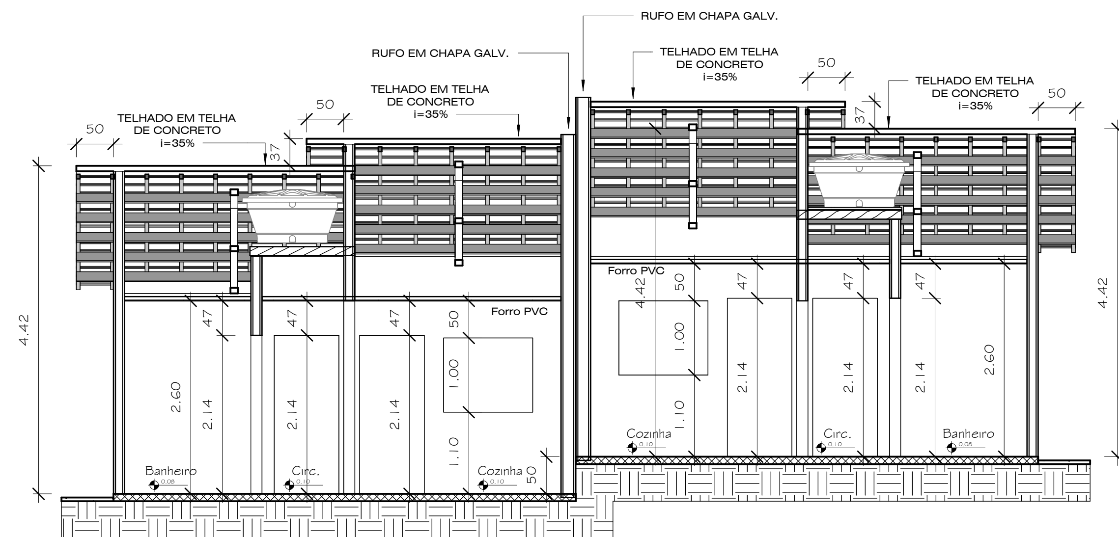
A Corte A 1 : 50
