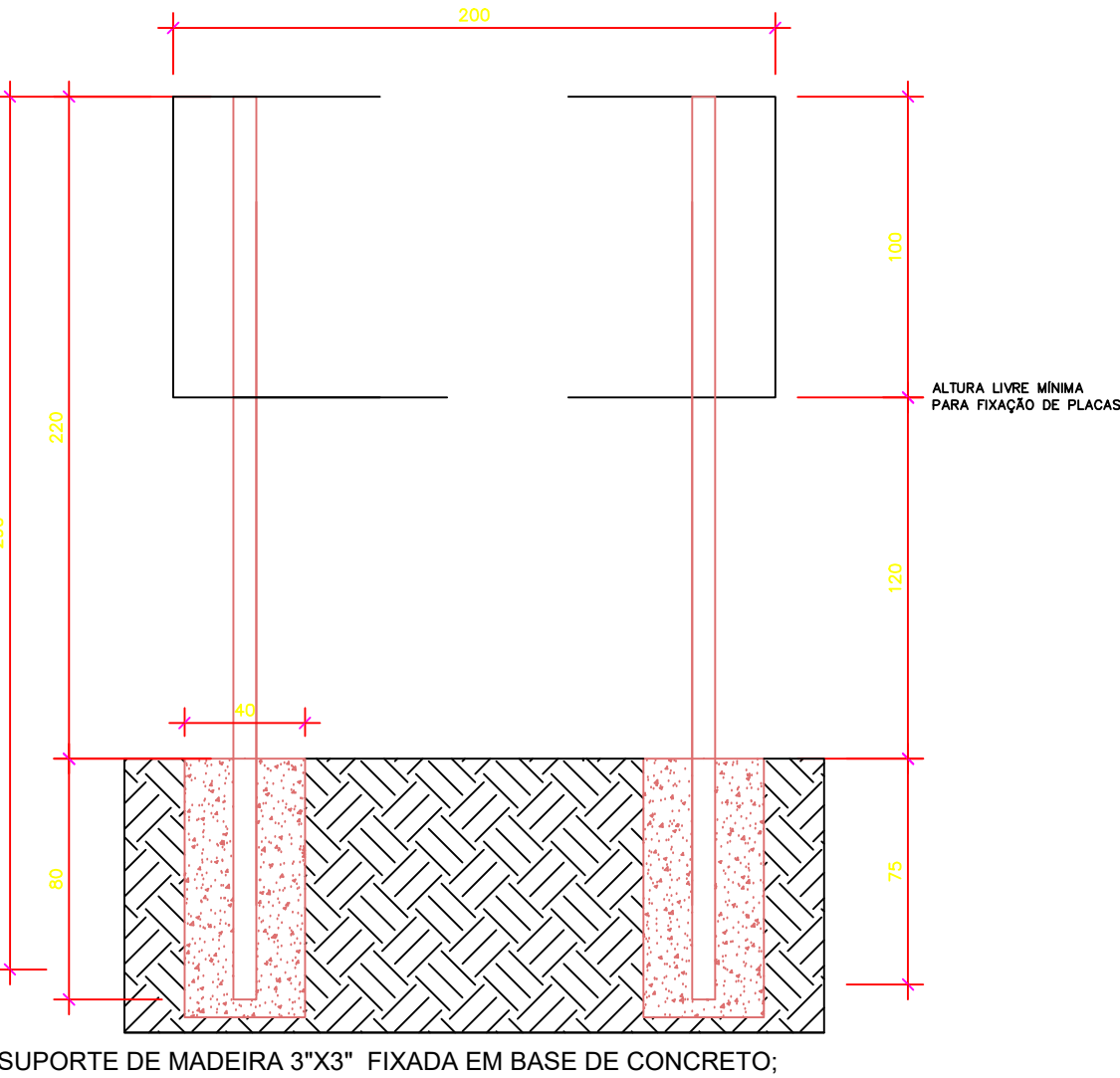
SUPORTE PARA PLACAS DE SINALIZAÇÃO – INDICAÇÃO
