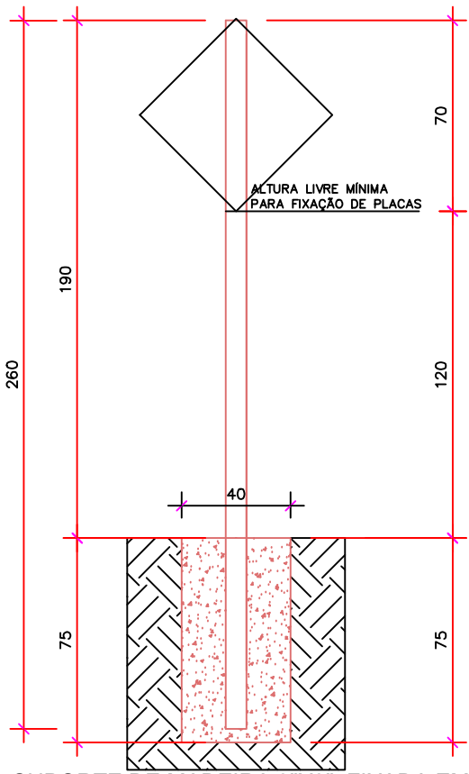
SUPORTE PARA PLACAS DE SINALIZAÇÃO
