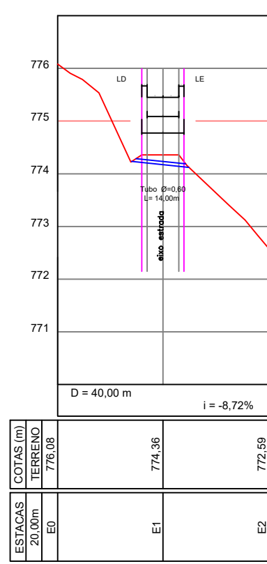
SEÇÃO TRANSVERSAL EST. 198
