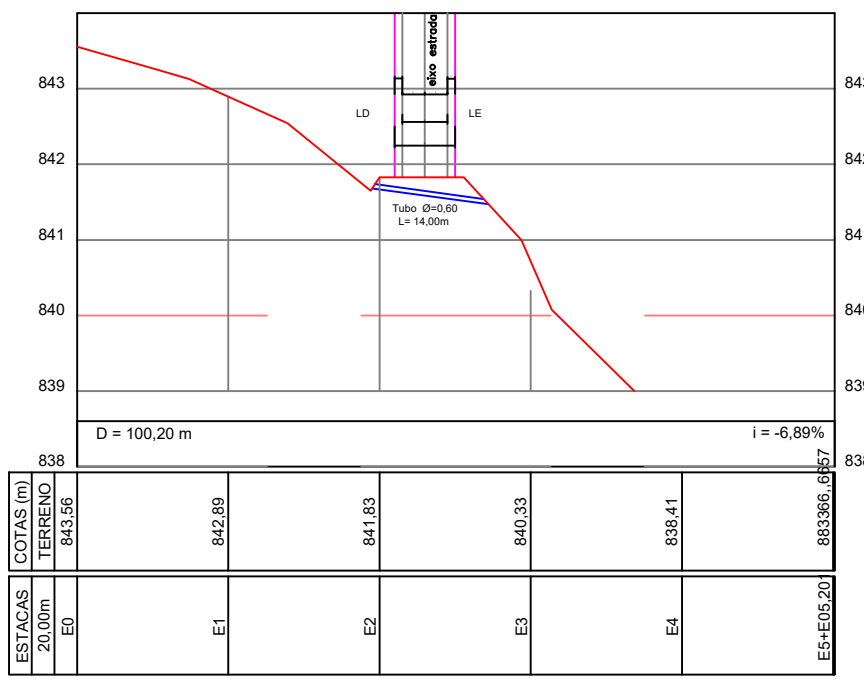
SEÇÃO TRANSVERSAL EST. 86
