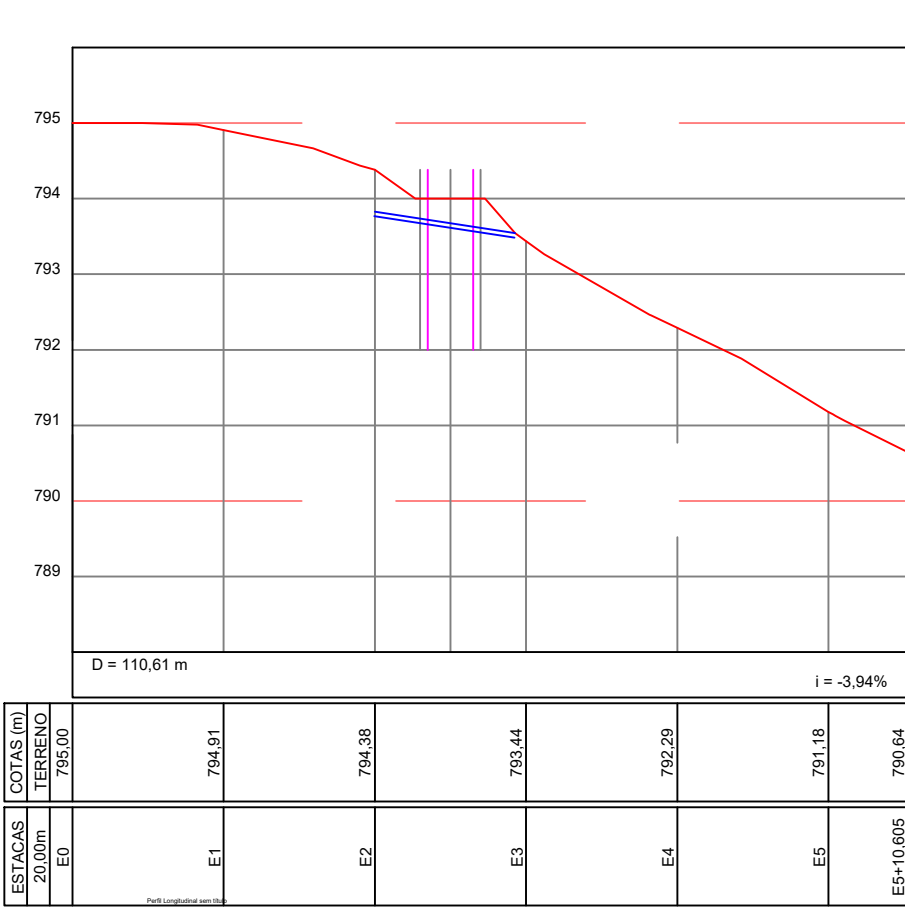
SEÇÃO TRANSVERSAL EST. 293
