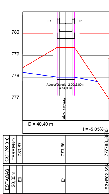
SEÇÃO TRANSVERSAL EST. 146
