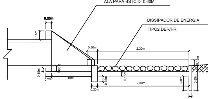
SECÇÃO LONGITUDINAL - DISSIPADOR
