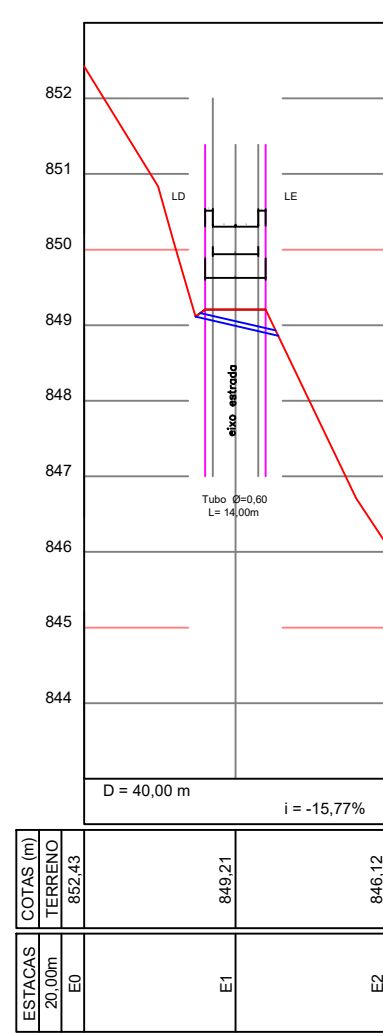
SEÇÃO TRANSVERSAL EST. 34
