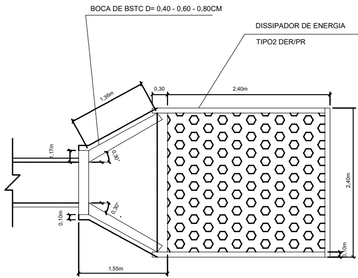
PLANTA - DISSIPADOR
