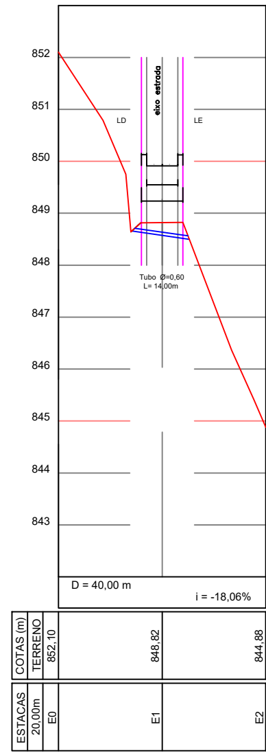
SEÇÃO TRANSVERSAL EST. 27
