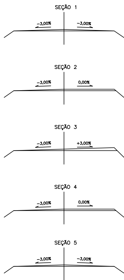
SUPERELEVÇÃO DE CURVA PARA A ESQUERDA
