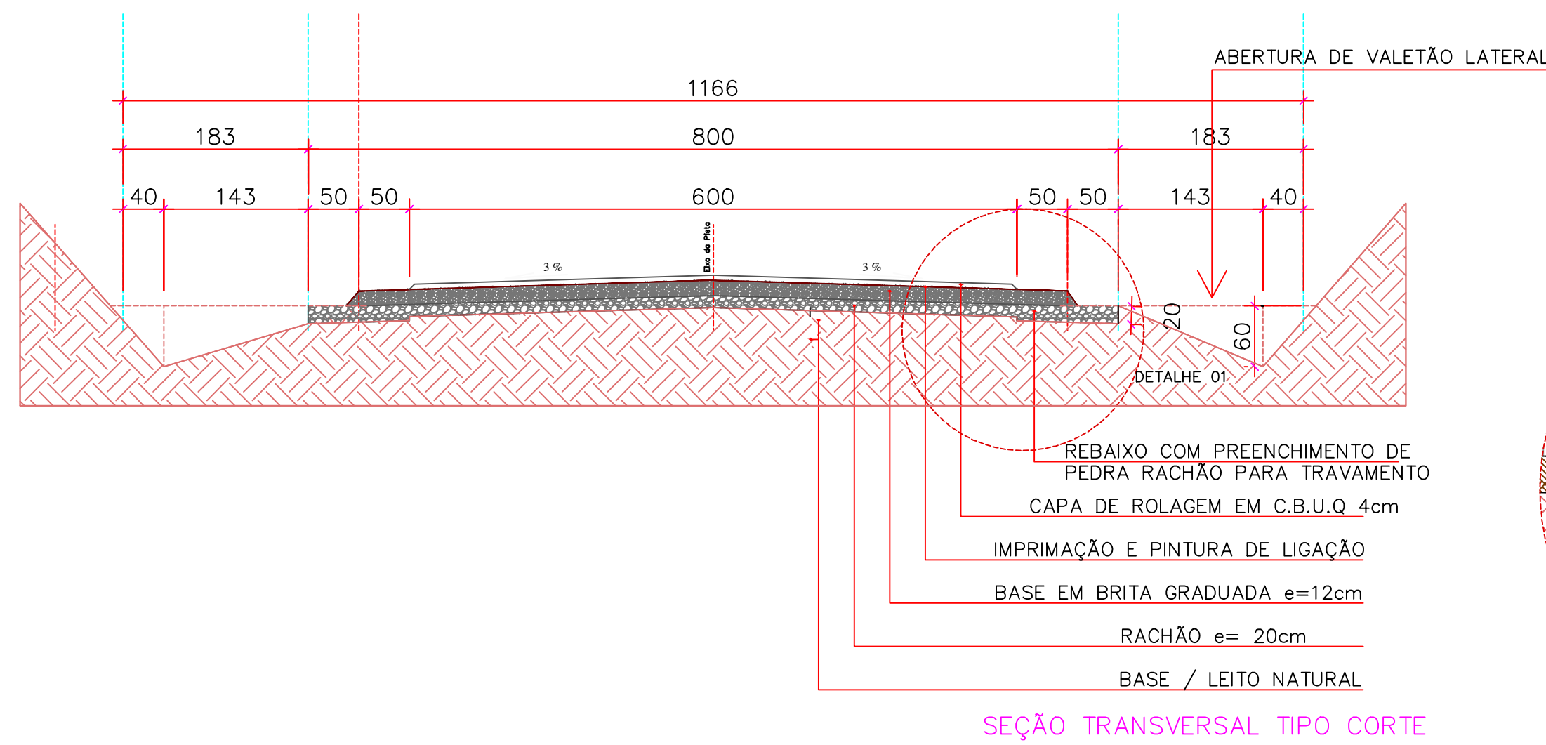
SEÇÃO TRANSVERSAL TIPO CORTE
