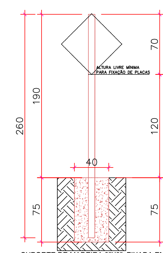
SUPORE PARA PLACAS DE SINALIZAÇÃO
