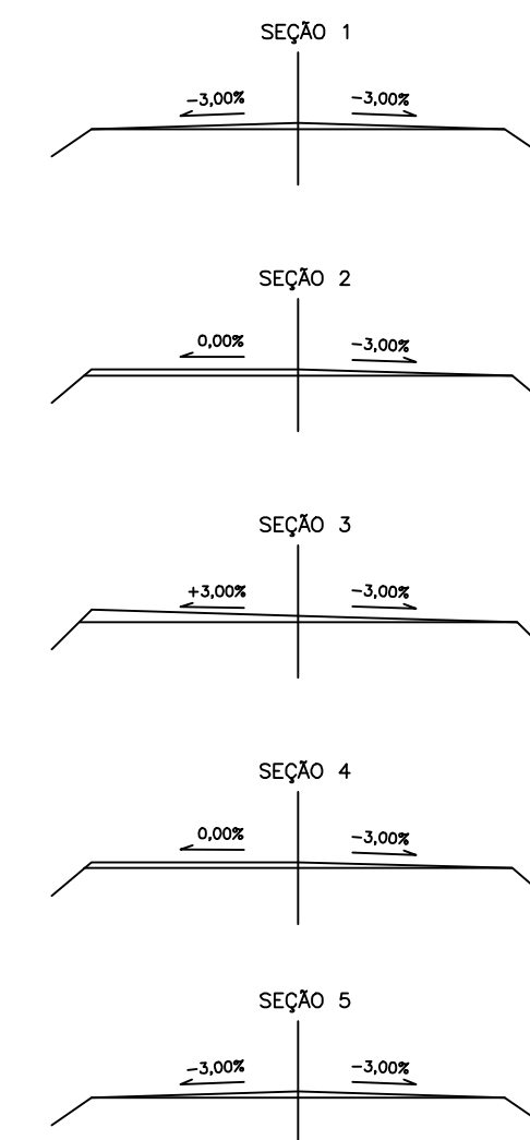
SUPERELEVÇÃO DE CURVA PARA A DIREITA
