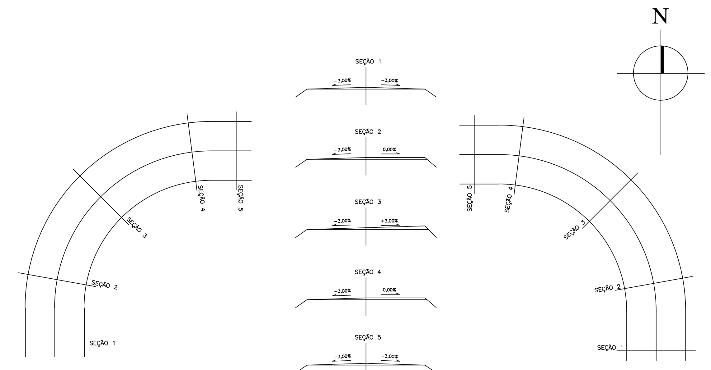
SUPERELEVÇÃO DE CURVA PARA A DIREITA
